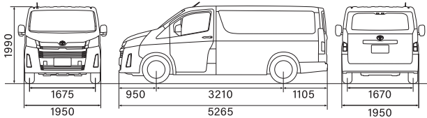
Carrocería estándar
